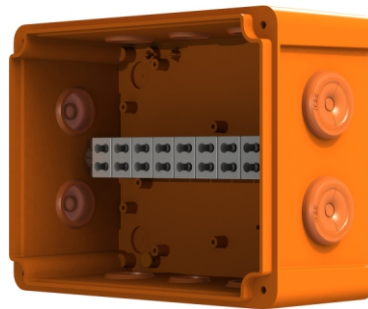
Klemmen horizontal
